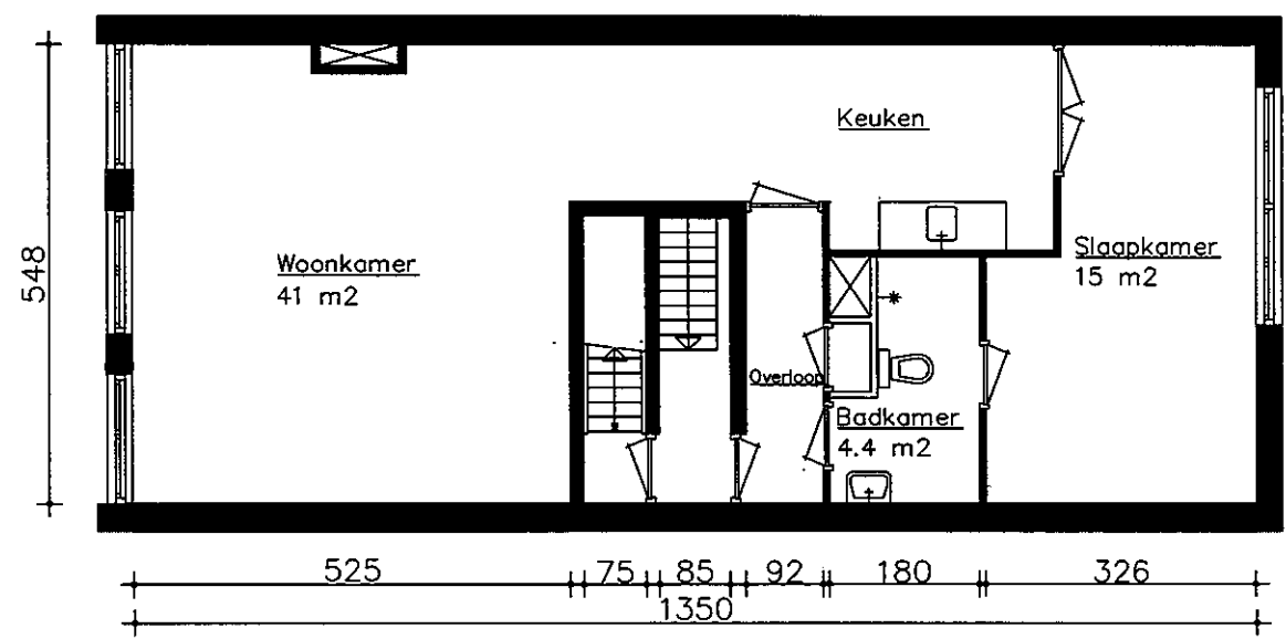
Tweede verdieping
